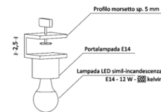
DETTAGLIO LAMPADINA CON MORSETTO
