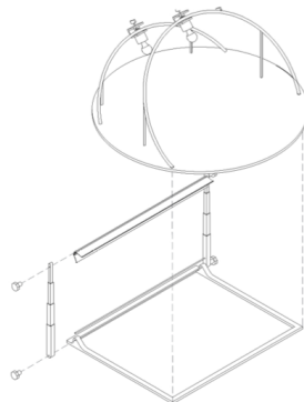
ASSONOMETRIA MONTAGGIO MAQUETTE SU SUPPORTO
