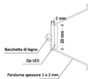
VISTA ASSONOMETRICA SUPPORTO
