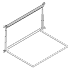
VISTA ASSONOMETRICA SUPPORTO
