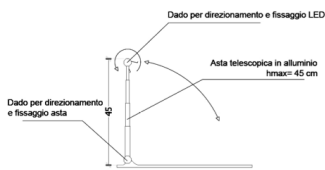
VISTA LATERALE SINISTRA SUPPORTO
