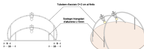
VISTA FRONTALE MAQUETTE M2C
